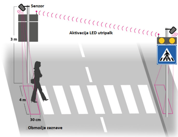
Shema postavitve sistema označitve prehoda za pešce Safety Cross
